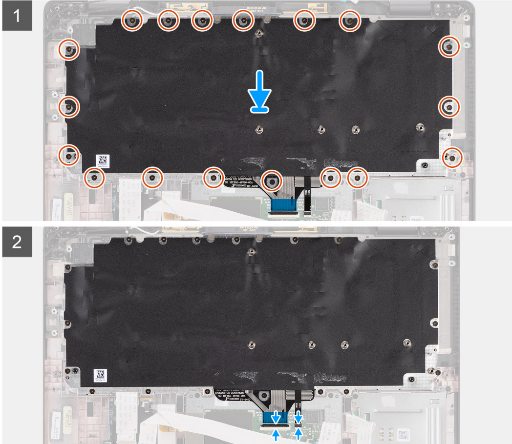
18x M1.6X1.7
